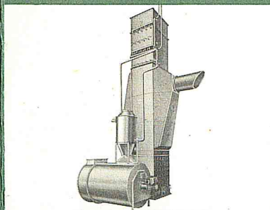
Kombinierter Warmluft- und Radiatoren- Körner Trockner Type Goldsaat KT-R 3/1 mit Luftheritzer WE 180
