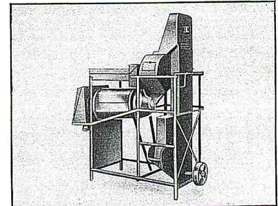
Beizmaschine »POPPELSDORF« geprüft und anerkannt. Leistung 250–1500 kg stündlich bei Schwergetreide
