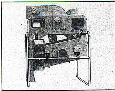
»GOLDSAAT«-Vorreiniger »G V«
