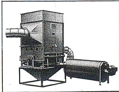
»GOLDSAAT«-Körnertrockner CONTINUS mit 500 kg Stundenleistung bei 4% Feuchtigkeitsentzug
