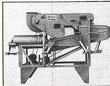
Saatgutbereiter »GOLDSAAT« 20/58 B. P. a. Stundenleistung 1000 kg/h Schwerfrucht-Aufschüttgut bei Saatgutherstellung
