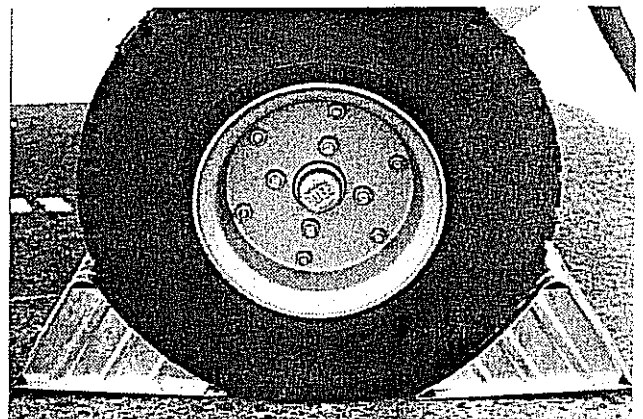
Bild 6: Sicherung der Räder bei ein- und zwei-achsigen Fahrwerken
