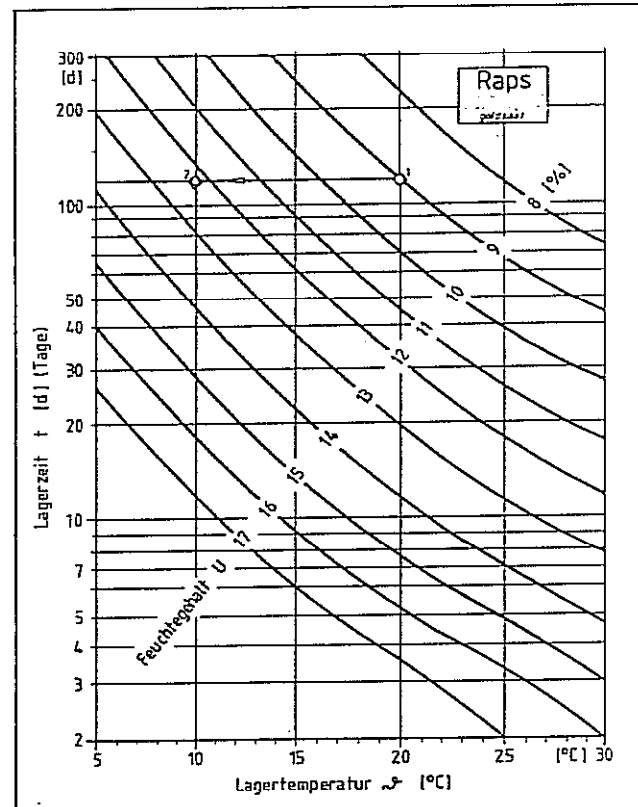
Bild 23: Lagerdauer von Raps in Abhängigkeit von Korntemperatur und -feuchte
