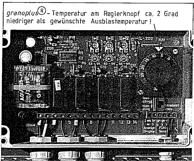
Bild 20: granoplus ® -Regelgerät im Schaltkasten (24)
