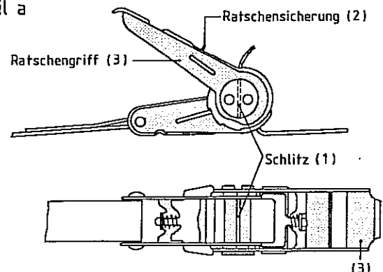
Bild 10: Kaltluftschlauch mit Spannratsche am Ausblasrohr (19) der Wechselplatte
