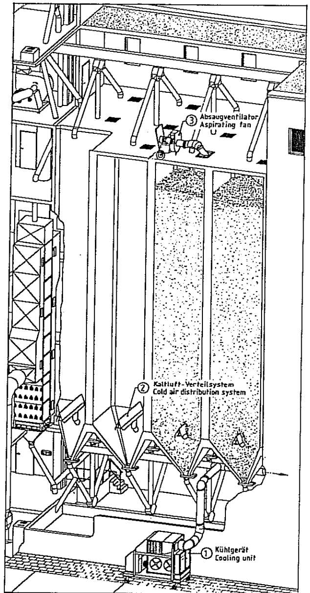
Bild 19: granosuc ® -Einrichtung zur Überwindung hoher Widerstände
