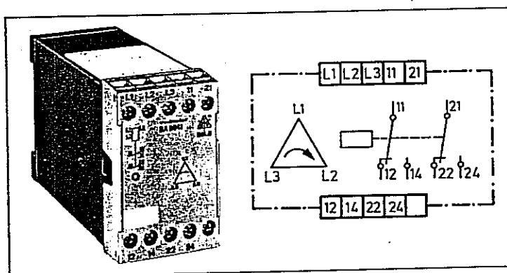
Bild 9: Phasenfolgerelais (BA) mit Schaltbild
